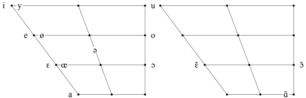
Figure 3. L'inventaire des voyelles du français supralocal
